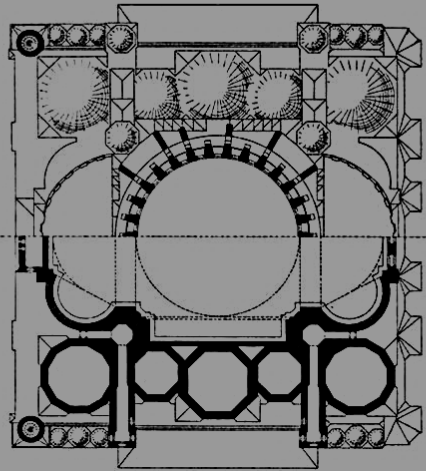
HORIZONTALSCHNITT DURCH DIE TAMBÜRE DER KLEINEN KUPPELN
